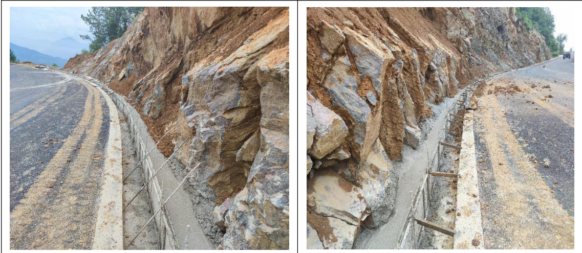
排水边沟支模
