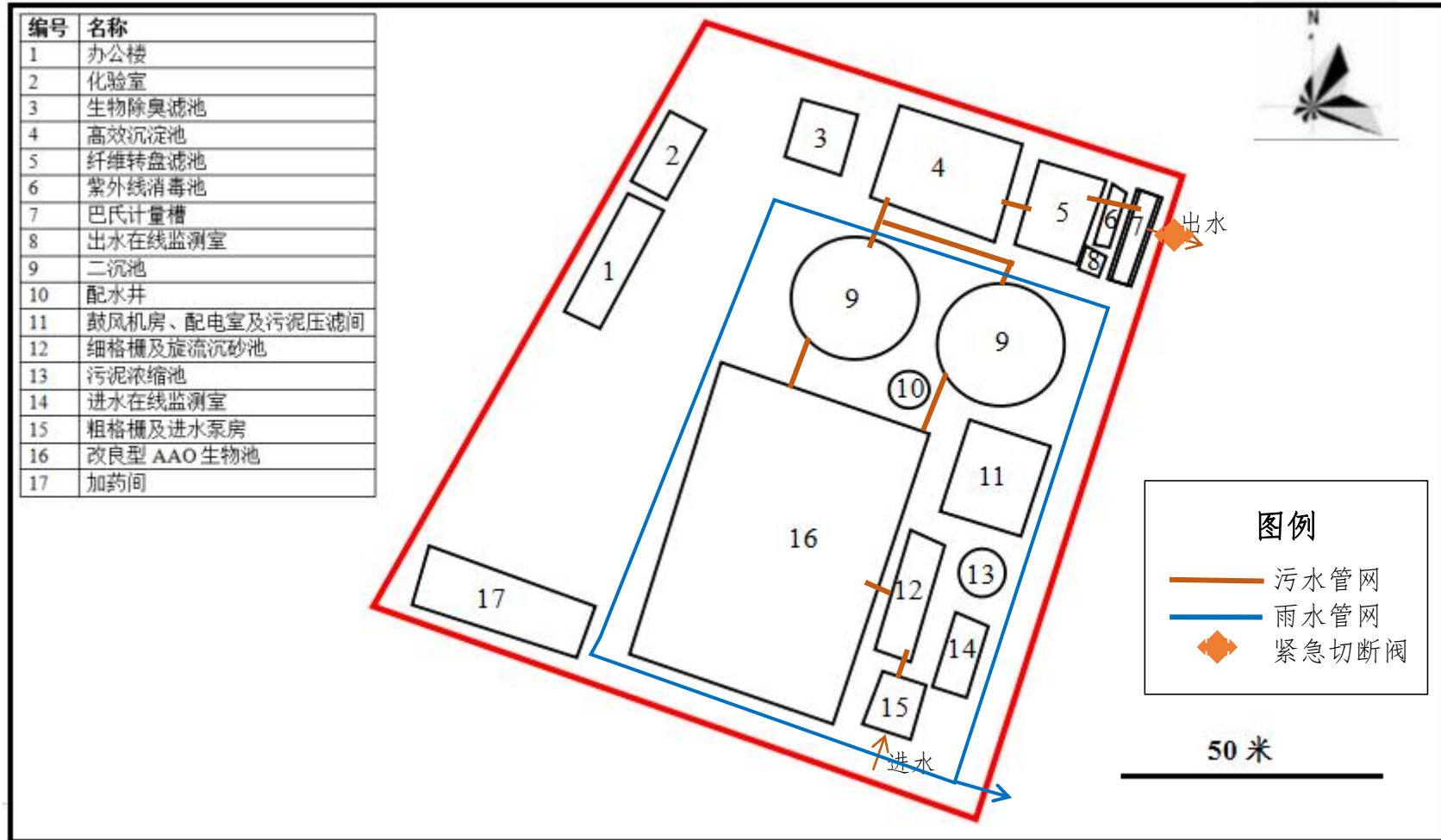
附件 4 宜都市城东污水处理厂雨污管网图
