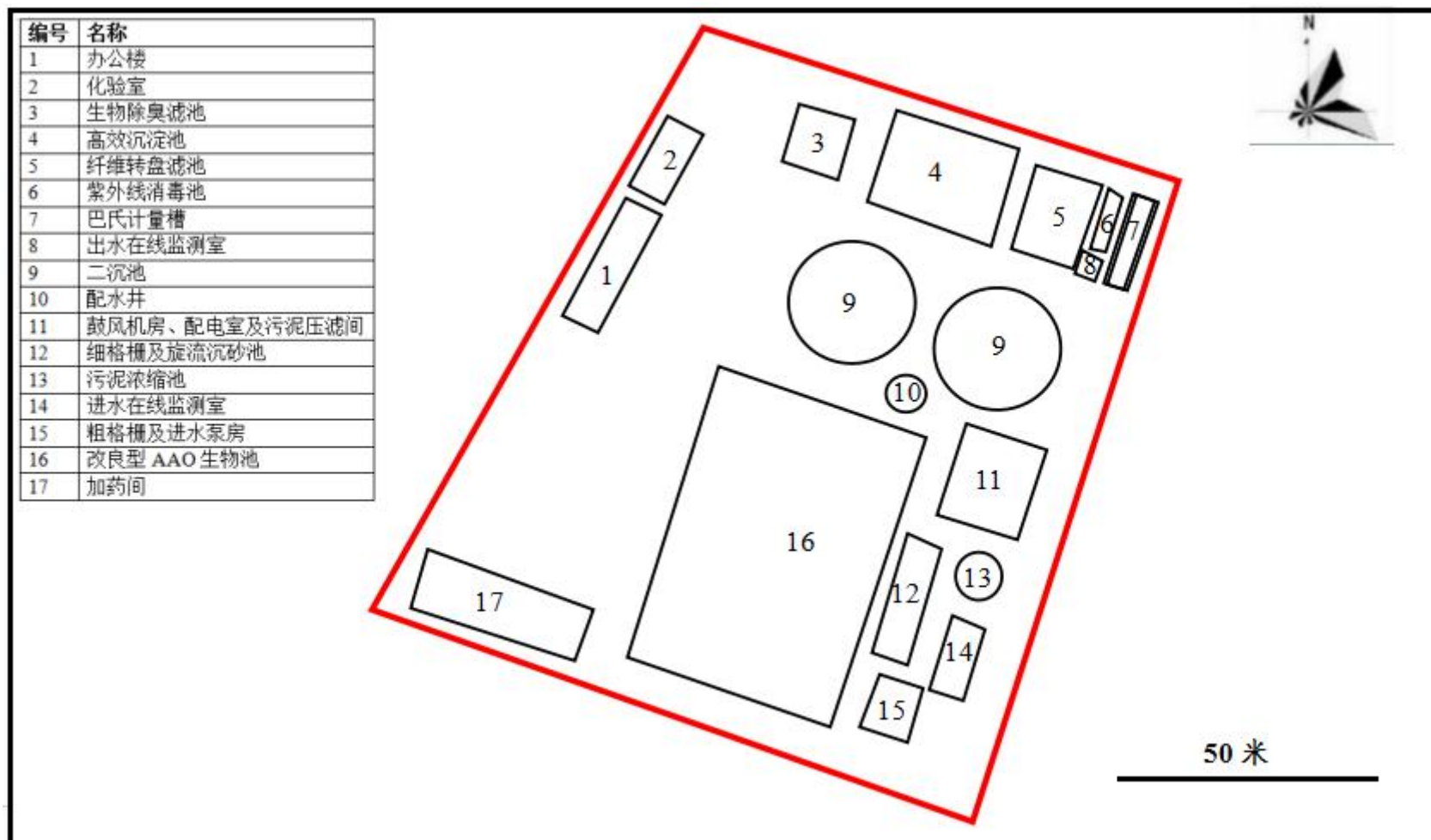
附件 2 宜都市城东污水处理厂平面布置图
