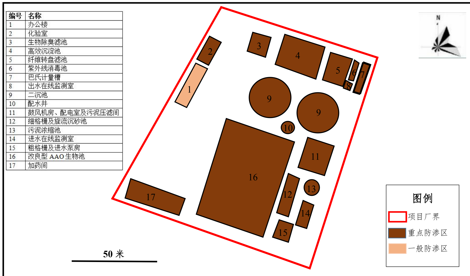
附件 8 宜都市城东污水处理厂分区防渗图
