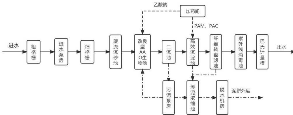
图 3-1 全厂工艺流程图
