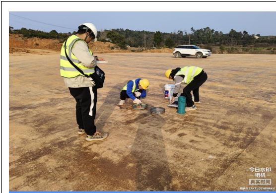
今日水印相机 真实时间 湖北省宜昌市峡州大道三期（杨家店……白洋）市政工程监理部 施工区 域: K15+180-240 施工内 容: 路基石方土质压实度检测 拍摄时 间: 2024.03.02 16:51:34 天 气: 晴 15℃ 地 点: 宜昌市·087步瀛 建设单位: 宜昌高新投资开发有限公司 监理单位: 中咨工程咨询有限公司 施工单位: 中国路桥集团第一工程有限公司 设计单位: 湖北省地质工程勘察院有限公司 勘察单位: 湖南化工地质工程勘察院有限公司 代建单位: 宜昌产投建设发展有限公司
