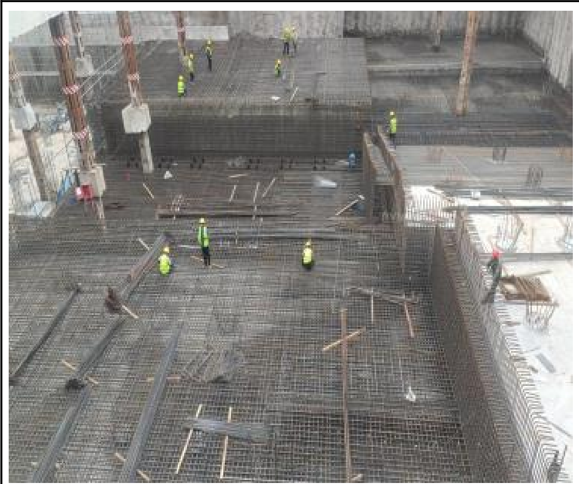
大公桥调蓄池主体结构钢筋绑扎
